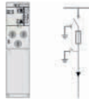
F – Sigortalı ayırıcı ve toprak bıçağı ünitesi 200A nominal akım, 5kA 1(s) kısa devre dayanım
