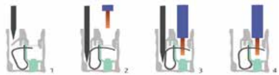
Yaylı Bağlantı
