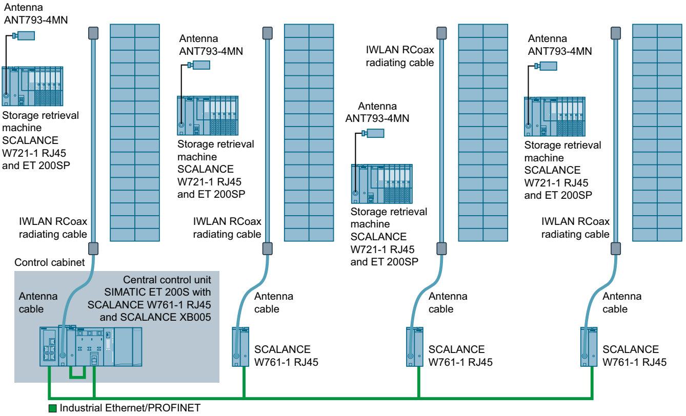
Rcoax kablosuz haberleşme sistemi örneği
